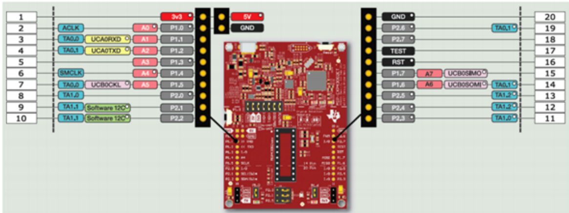
Figure 19 - MSP430G2ET [28]
